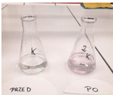
Zabarwienie przesącza przed (przesącz bezbarwny, klarowny) i po miareczkowaniu (przesącz lekko różowy, klarowny)
